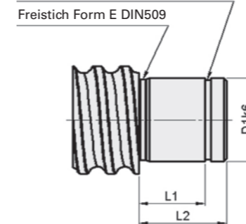
Einstich für Sicherungsring DIN471
